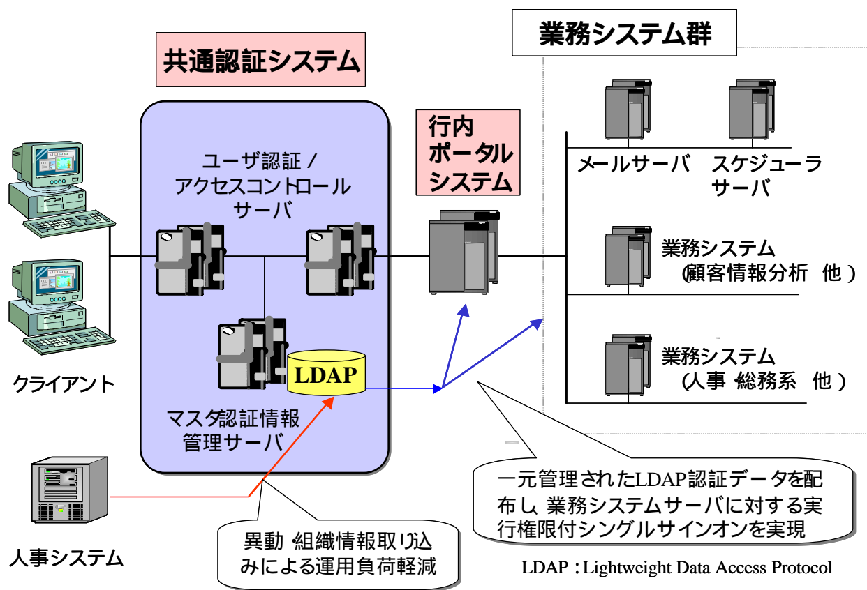
共通認証システムとポータルシステム連携概要構成図
